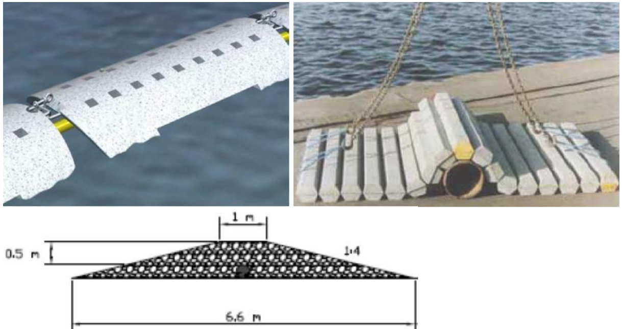
Figur 4.6. Mekanisk beskyttelse av kabel med betongprofil (øverst t.v), betongmadrass (øverst t.h) og steinfylling (nederst).
